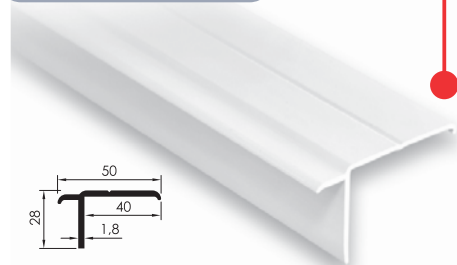
T Profil 10x40 (Everest)
