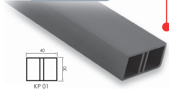
Kutu Profil (Siding)
