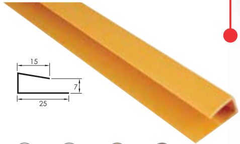
U Profil
