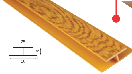
H Profil
