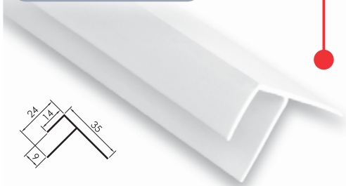
F Profil
